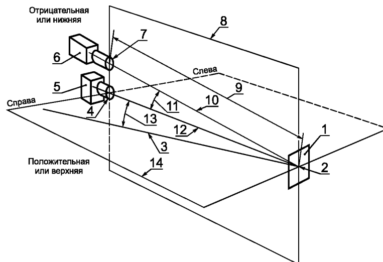
Установка оборудования для испытания световозвращателя
