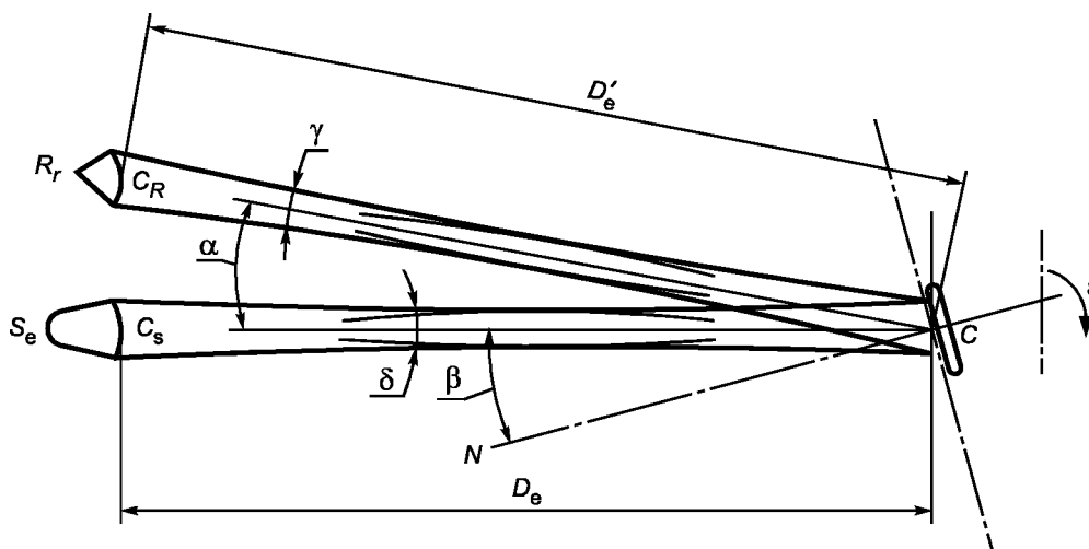
Схема для пояснения используемых обозначений
