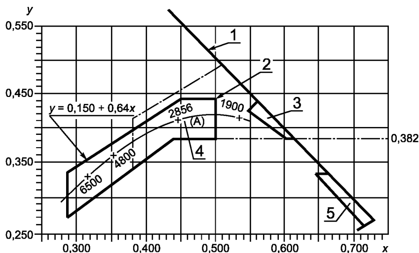
Границы световых участков для световозвращающих устройств
