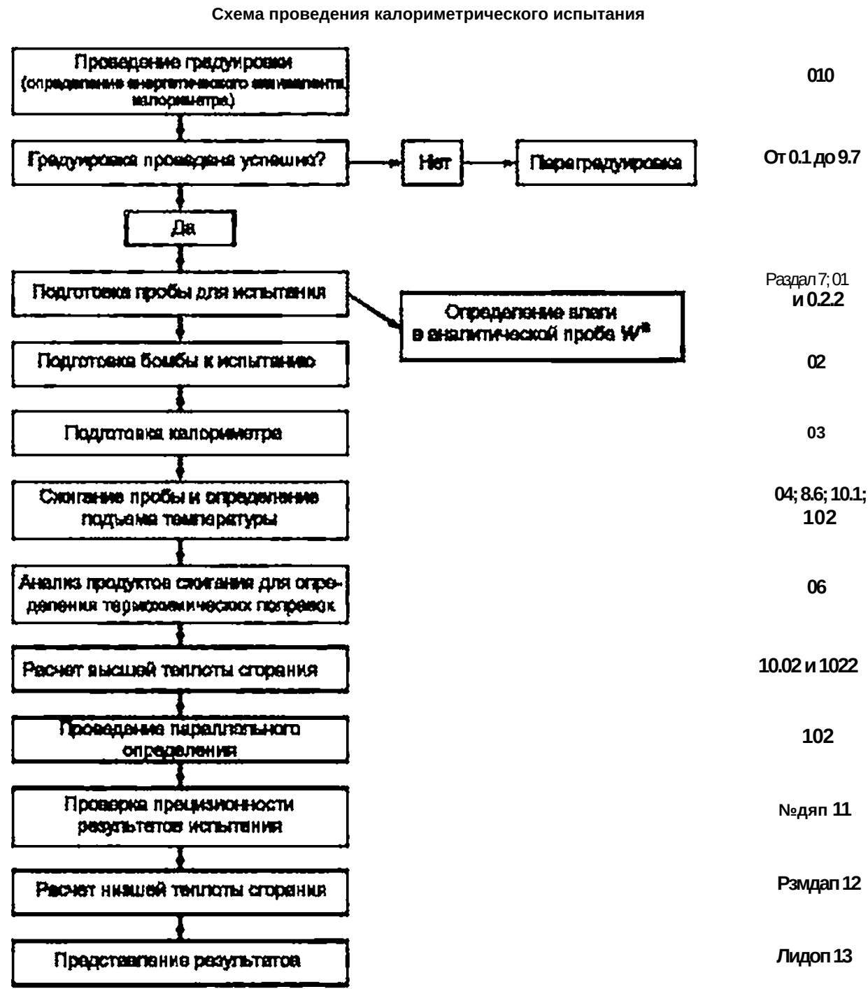
Рисунок G.1 — Схема рядового калориметрического испытания
