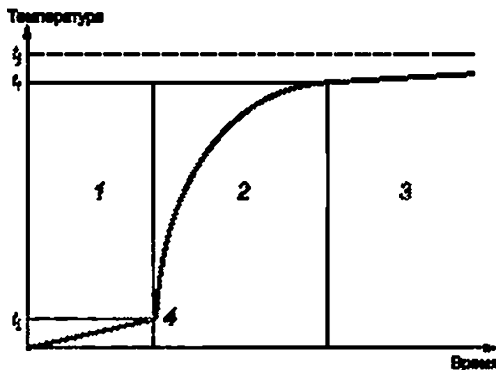
4 — начальная температура главного периода; t_f — конечная температура главного периода; t_l — температура термостата (кожуха); 1 — начальный период; 2 — главный период; 3 — конечный период; 4 — зажигание
