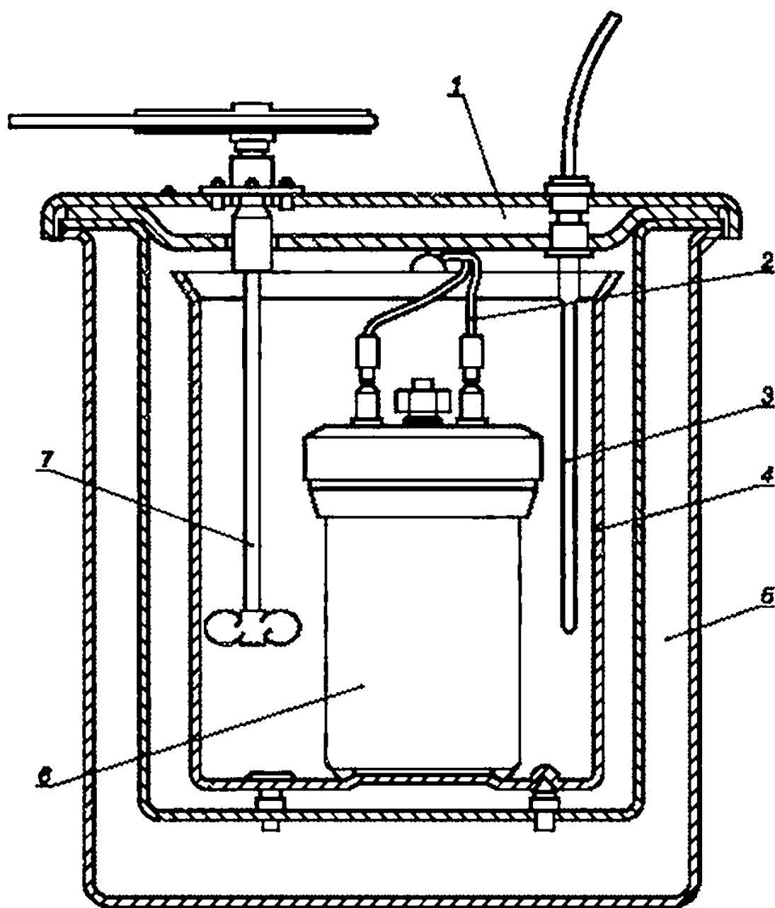
t — крышка термостата. 2 — контактные проходы системы зажигания. 3 — термометр. 4 — калориметрический сосуд. 5 — термостат; в — калориметрическая бомба; 7 — мешалка
