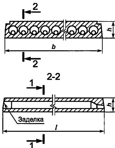
Рисунок 2 — Поперечные сечения плиты
