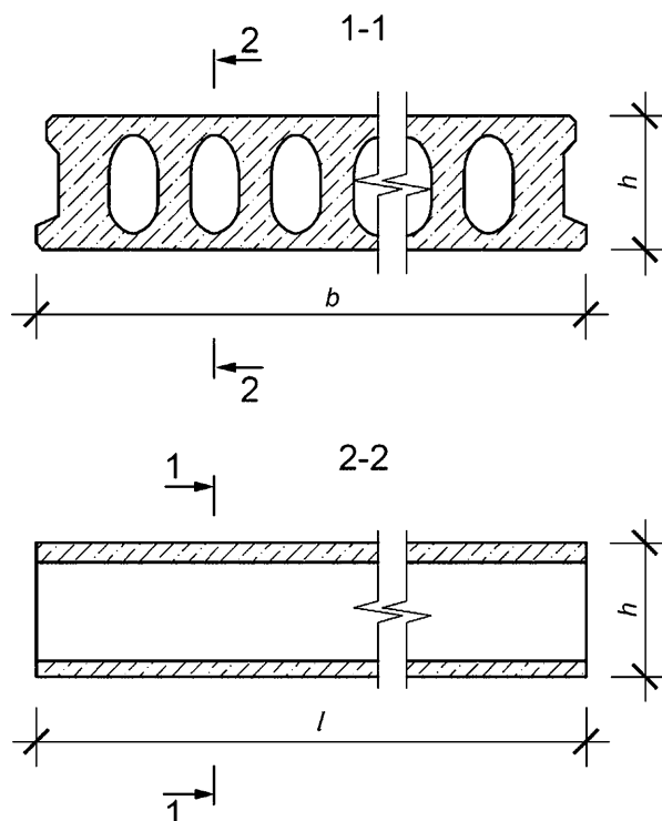
Рисунок 4 — Пример сечения плиты типа ПБ».
