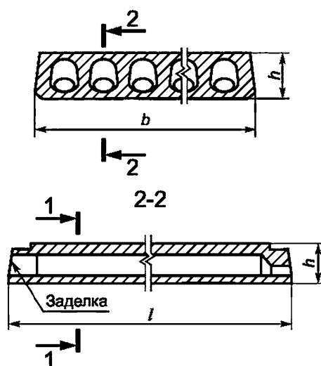
Рисунок 3 — Поперечные сечения плиты
