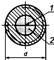
1 — ось крепежного изделия; 2 — область половины радиуса сечения (радиус 0.254)
