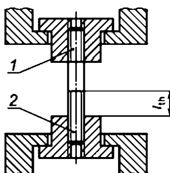
в) Пример испытательного устройства для шпилек
