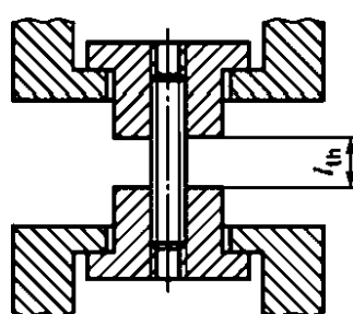
г) Пример испытательного устройства для шпилек с резьбой по всей длине
