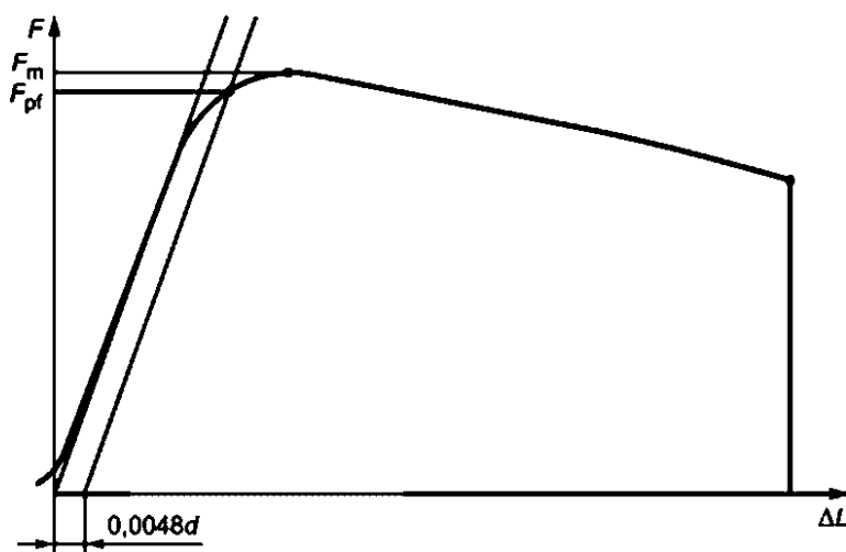
Рисунок 4 — Диаграмма нагрузка — перемещение для определения условного предела текучести при остаточном удлинении 0,00480
