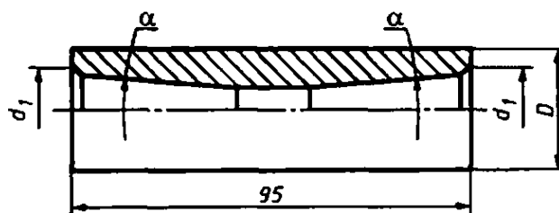
Рисунок 3 — Соединительная муфта
