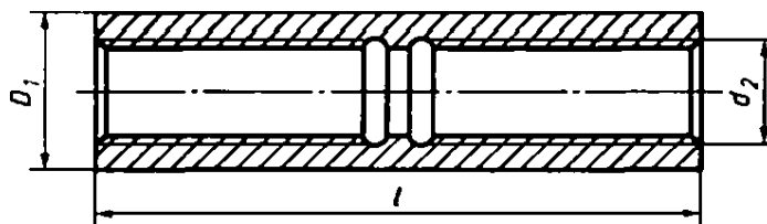
Рисунок 6 — Соединительная муфта
