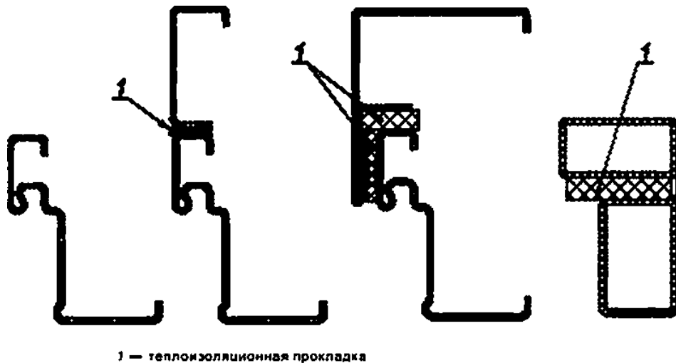
Рисунок Б.1 — Примеры конструктивного исполнения дверных коробок
