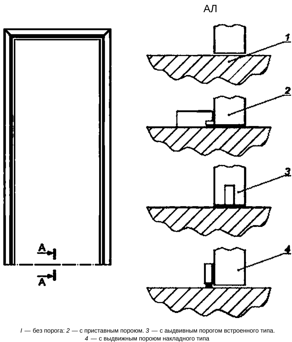
Рисунок А.5 — Примеры конструктивного исполнения дверей с «Г»-образной (незамкнутой) коробкой
