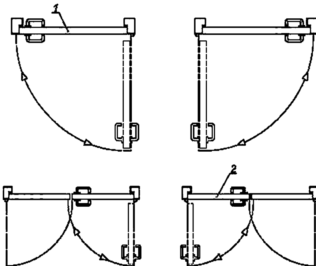
Рисунок А.3 — Примеры направления открывания дверей
