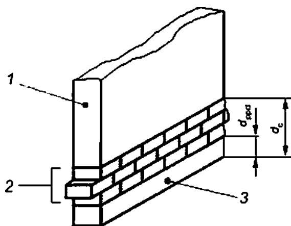
Рисунок 1 — Перемычка заводского изготовления (см. 3.1.19)
