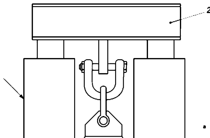
1 — гидравлический или механический силовой цилиндр; 2 — узкополочная двутавровая балка с опорой проушины
