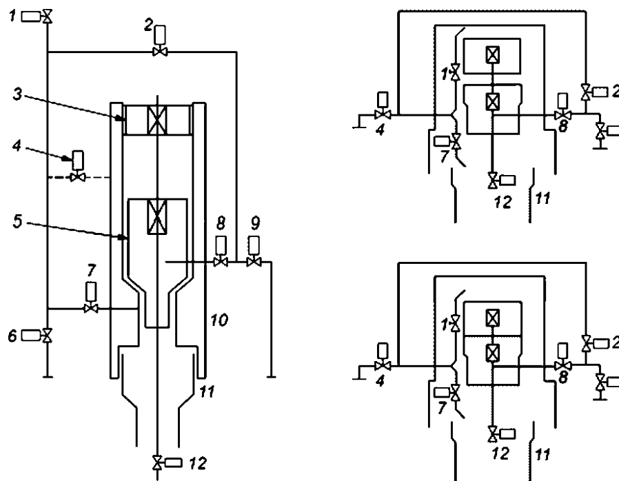
Рисунок 2 — Пример устьевых елок вертикального типа, смонтированных на устьевых трубных головках
