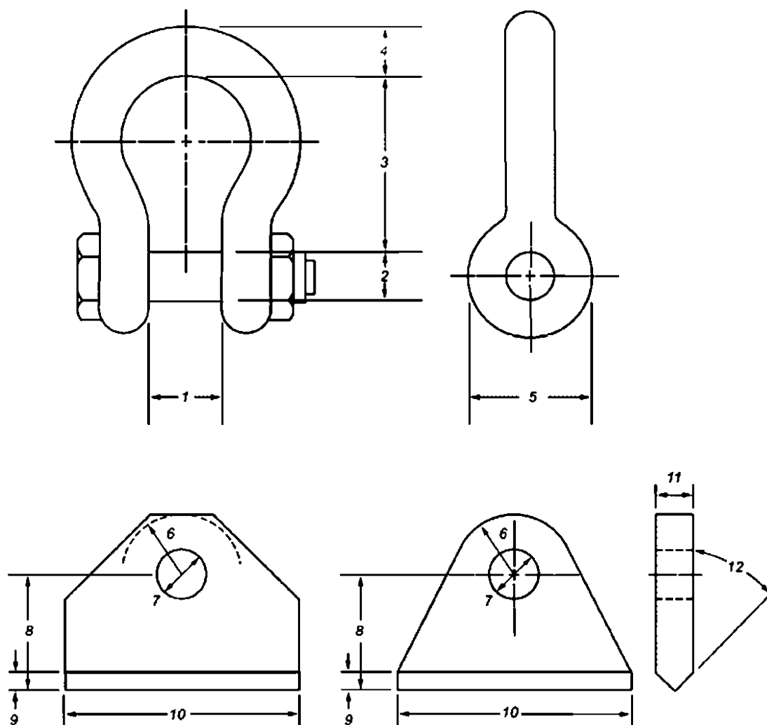
1 — ширина захвата серьги A , 2 — диаметр пальца серьги B ; 3 — внутренняя длина серьги C ; 4 — толщина проушины серьги N ; 5 — ширина фланца серьги F ; 6 — минимальное расстояние от центра отверстия под палец до кромки проушины J ; 7 — диаметр отверстия H ; 8 — расстояние от основания до центра отверстия проушины H ; 9 — толщина сварного шва проушины, равная t/h для швов с проплавлением h ; 10 — длина проушины L ; l_f — толщина проушины G ; 12 — угол схода кромки для подготовки к сварке p
