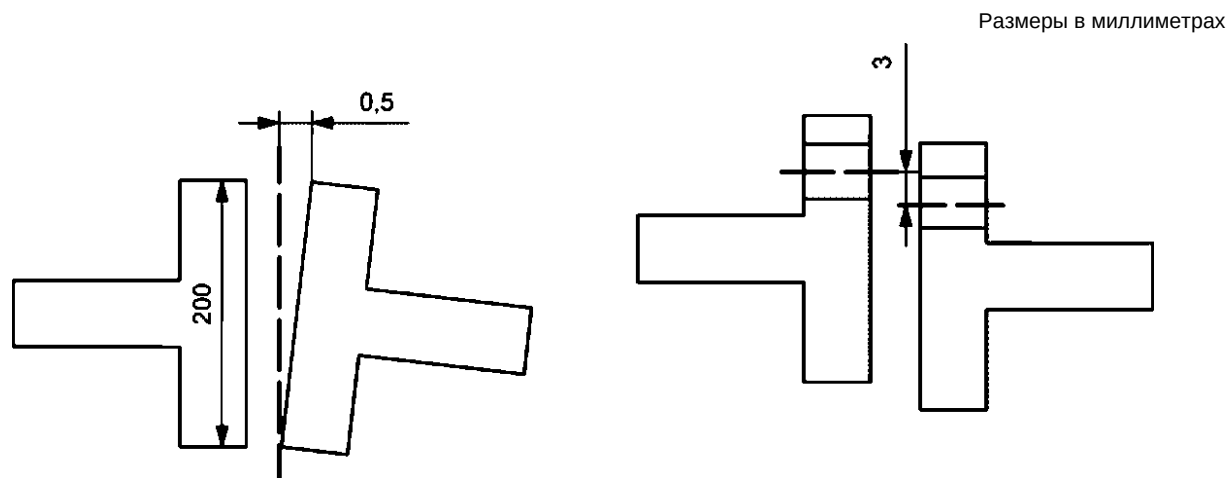
Рисунок G.1 — Допуски выравнивания фланцев
