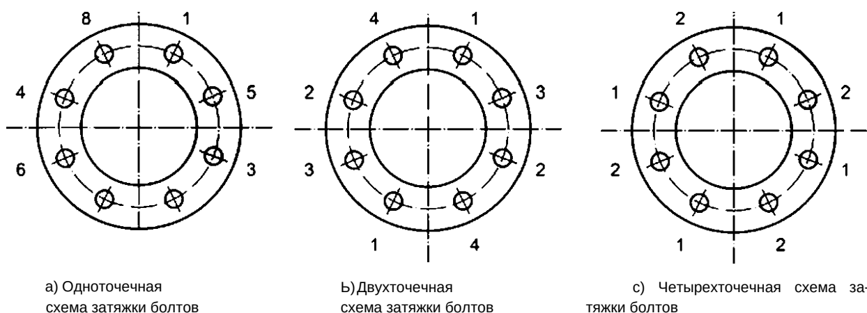
Рисунок G.2 — Перекрестная последовательность затяжки болтов одним, двумя и четырьмя инструментами одновременно
