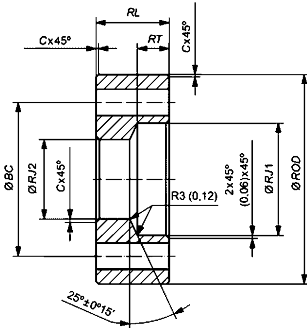
Базовые размеры тарелки*)
