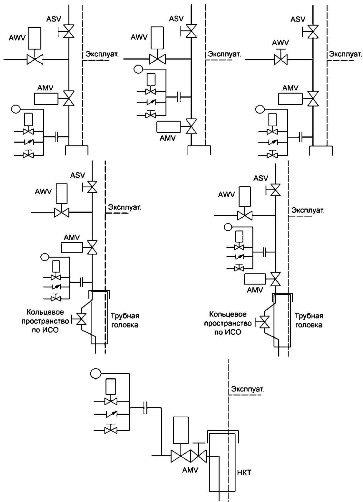
Б) Примеры проходок (пенетраций) кольцевых каналов
