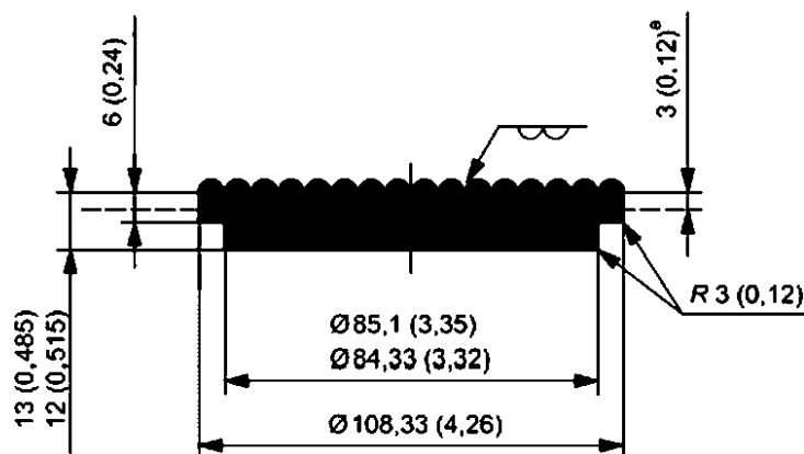
Рисунок 7 — Альтернативная детализация черновой и финишной машинной обработки для коррозионно-стойких кольцевых канавок 8X-149 и BX-150
