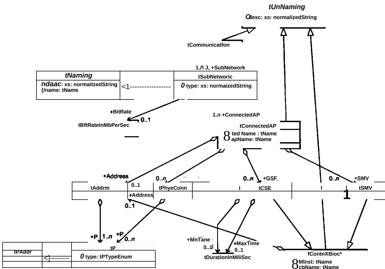
Рисунок 16 — Общее представление о секции Communication через схему UML
