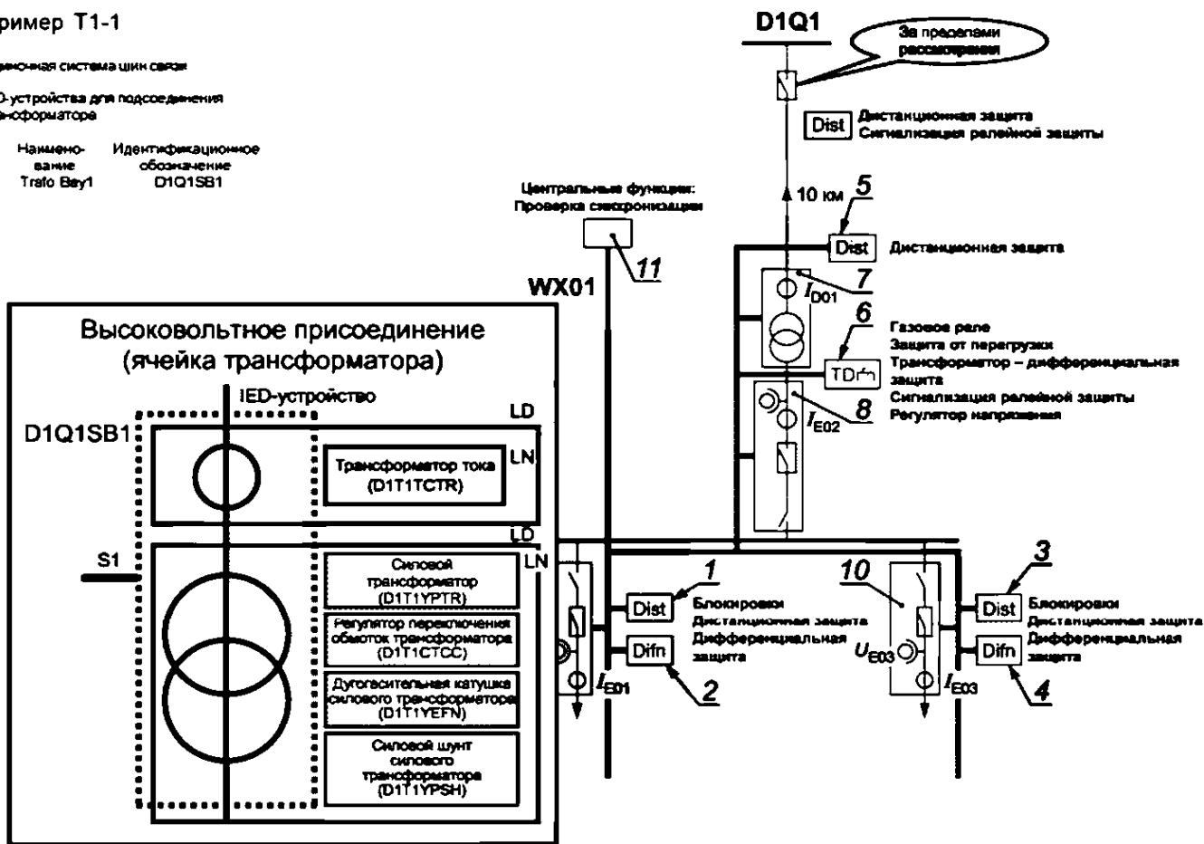
Рисунок D.3 — Ячейка трансформатора T1-1
