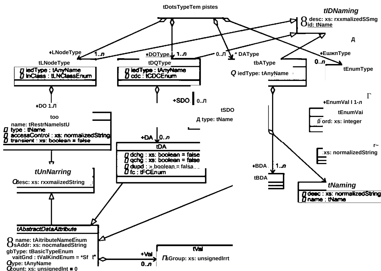
Рисунок 17 — Общее представление о секции DataTypeTemplates на основе UML
