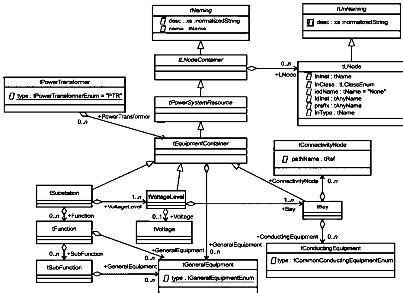
Рисунок 10 — UML-схема секции Substation
