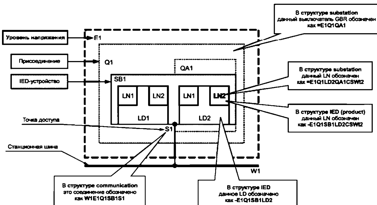
Рисунок 8 — Имена в различных структурах объектной модели
