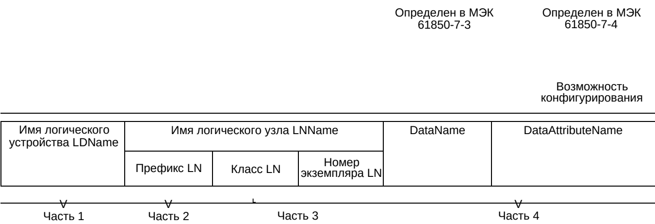
Рисунок 5 — Элементы идентификации сигнала согласно определению МЭК 61850-7-2
