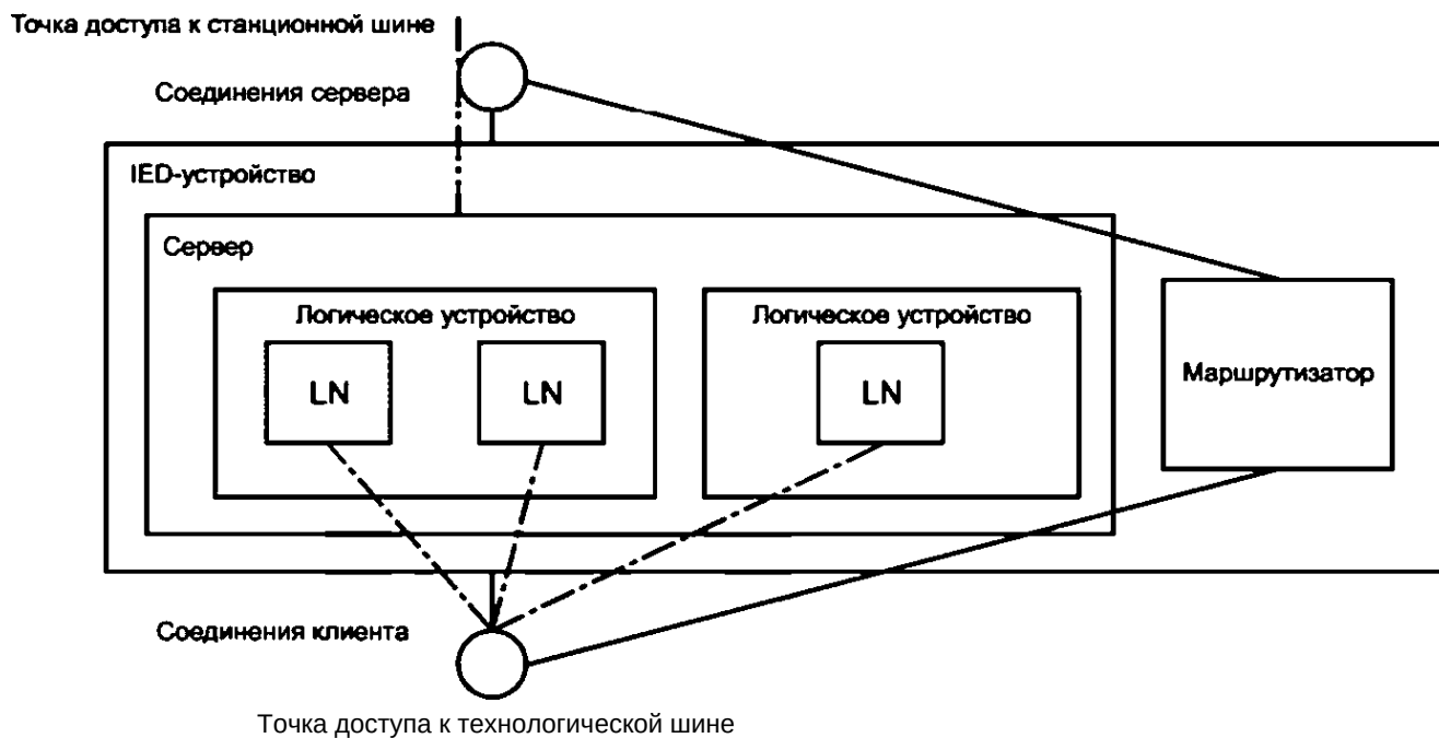
Рисунок 12 - Структура IED-устройства и точки доступа
