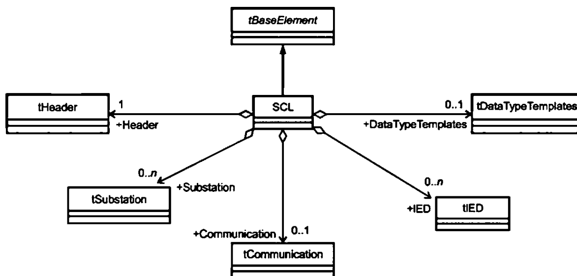
Рисунок 4 — Общее представление о схеме SCL в виде схемы UML
