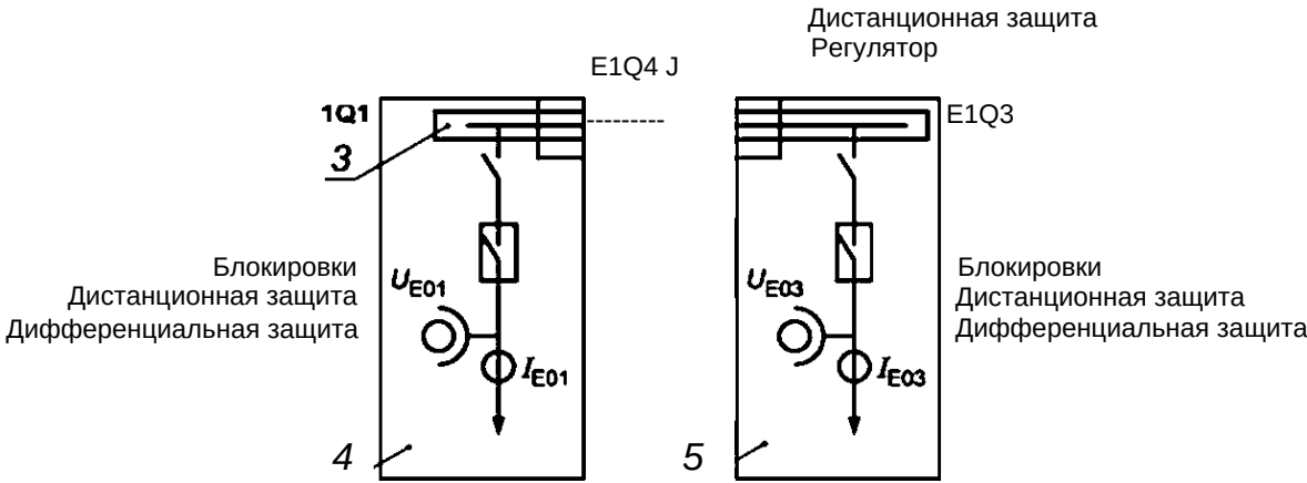
Рисунок D.1 — T1-1. Конфигурация подстанции
