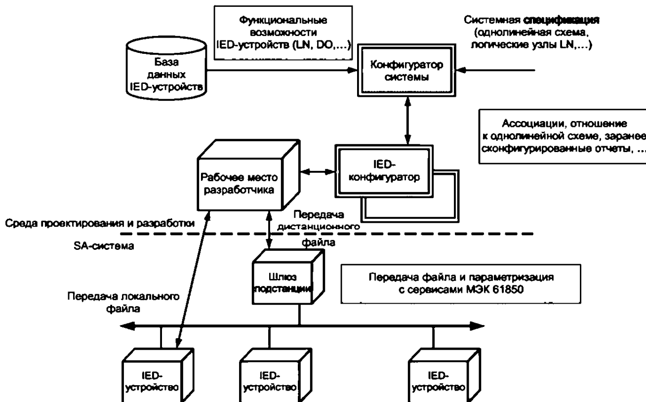
Рисунок 1 — Эталонная модель потока информации в процессе конфигурирования
