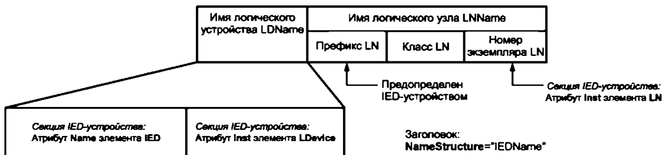
Рисунок 7 — Элементы имени сигнала при продукт-зависимом присвоении имени
