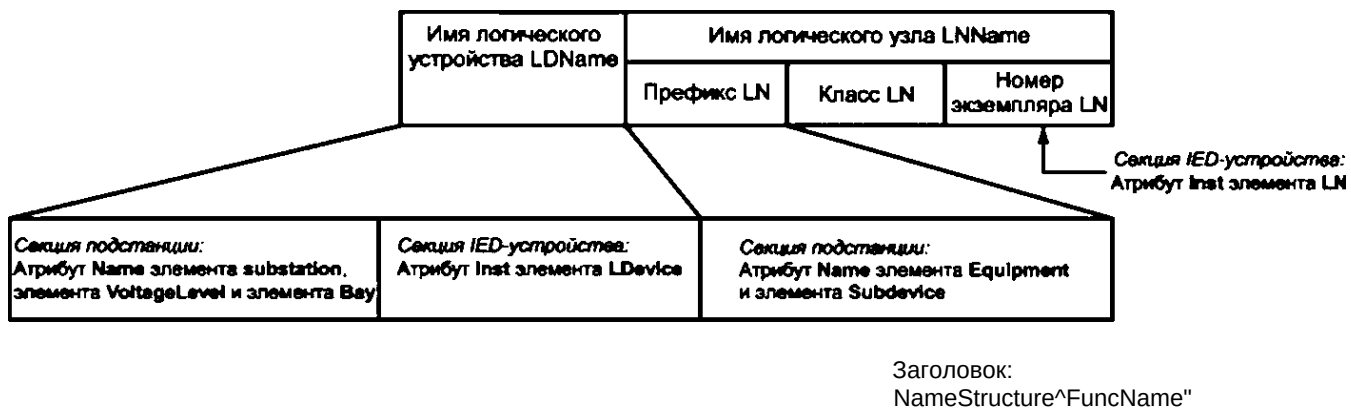
Рисунок 6 — Элементы имени сигнала при функциональном присвоении имен
