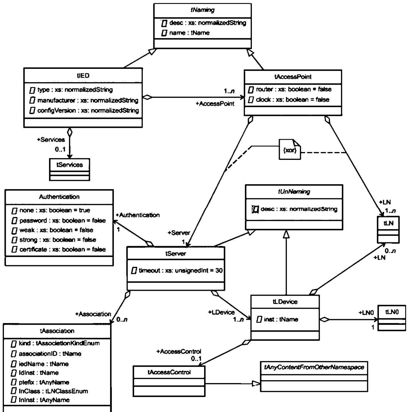
Рисунок 13 — UML-описание части схемы, относящейся к IED-устройству, — база
