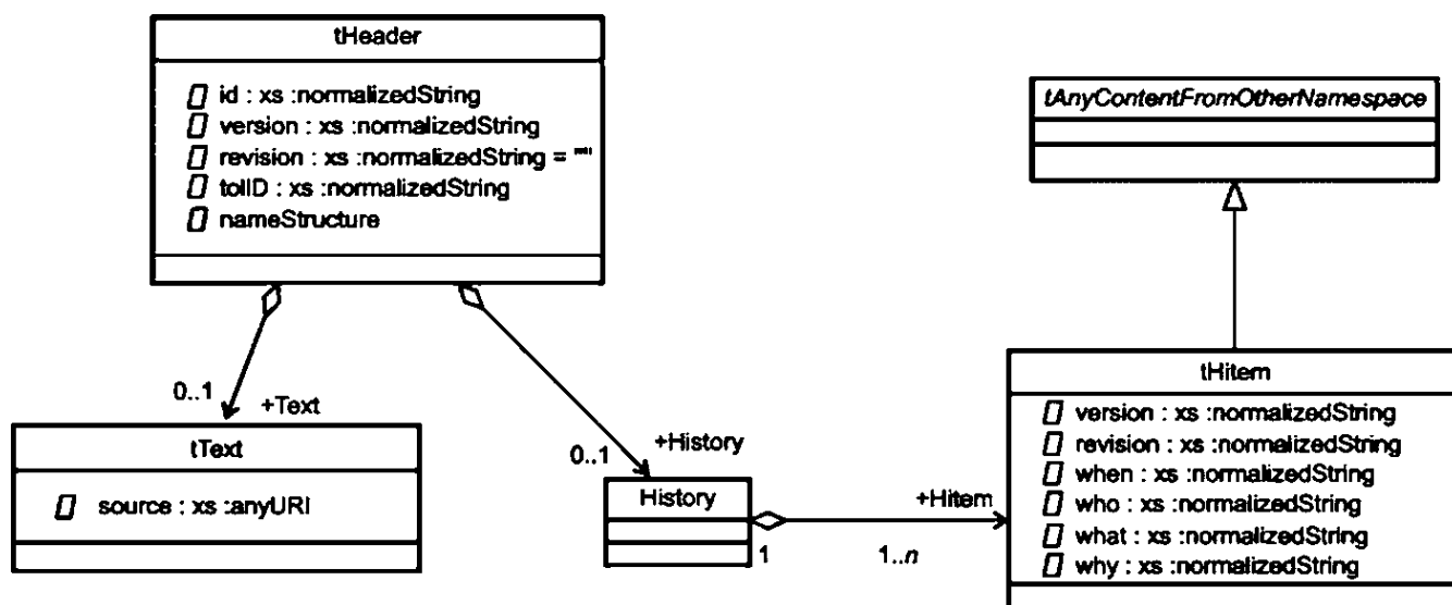
Рисунок 9 — UML-схема секции Header
