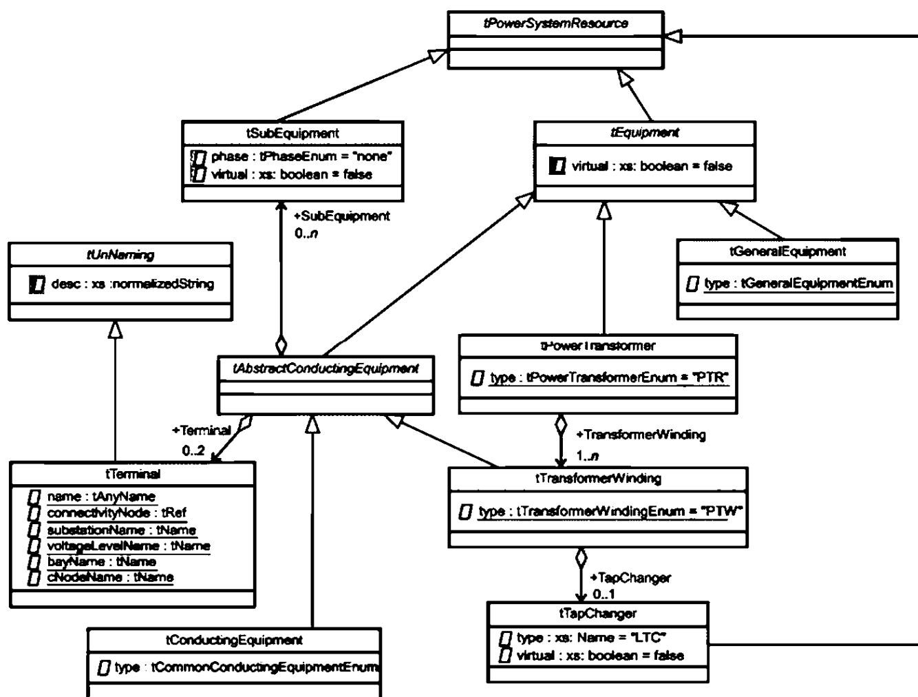
Рисунок 11 — UML-схема. Наследование типов оборудования и отношения
